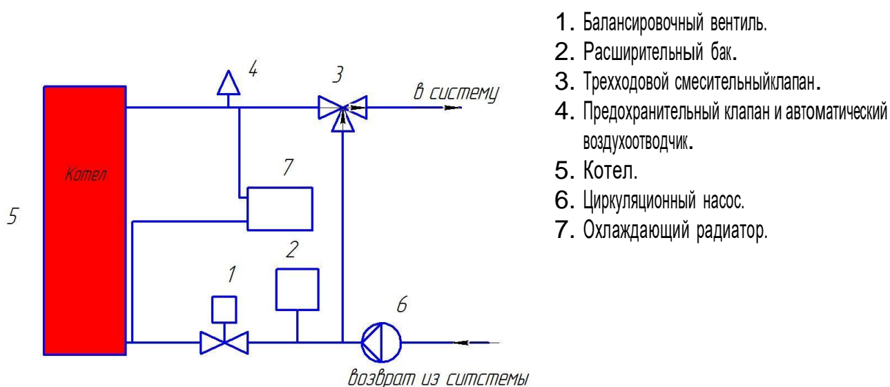
Рис.4. Принципиальная схема узла с подключением бойлера, безтеплых полов.
