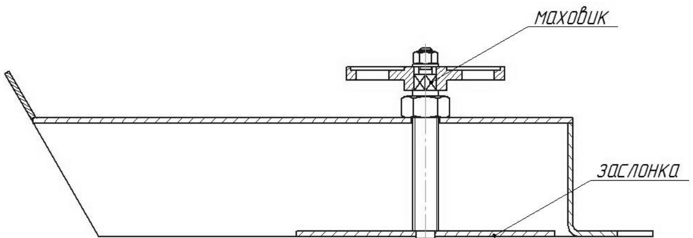
Рис.11 Регулятор подачи воздуха.
