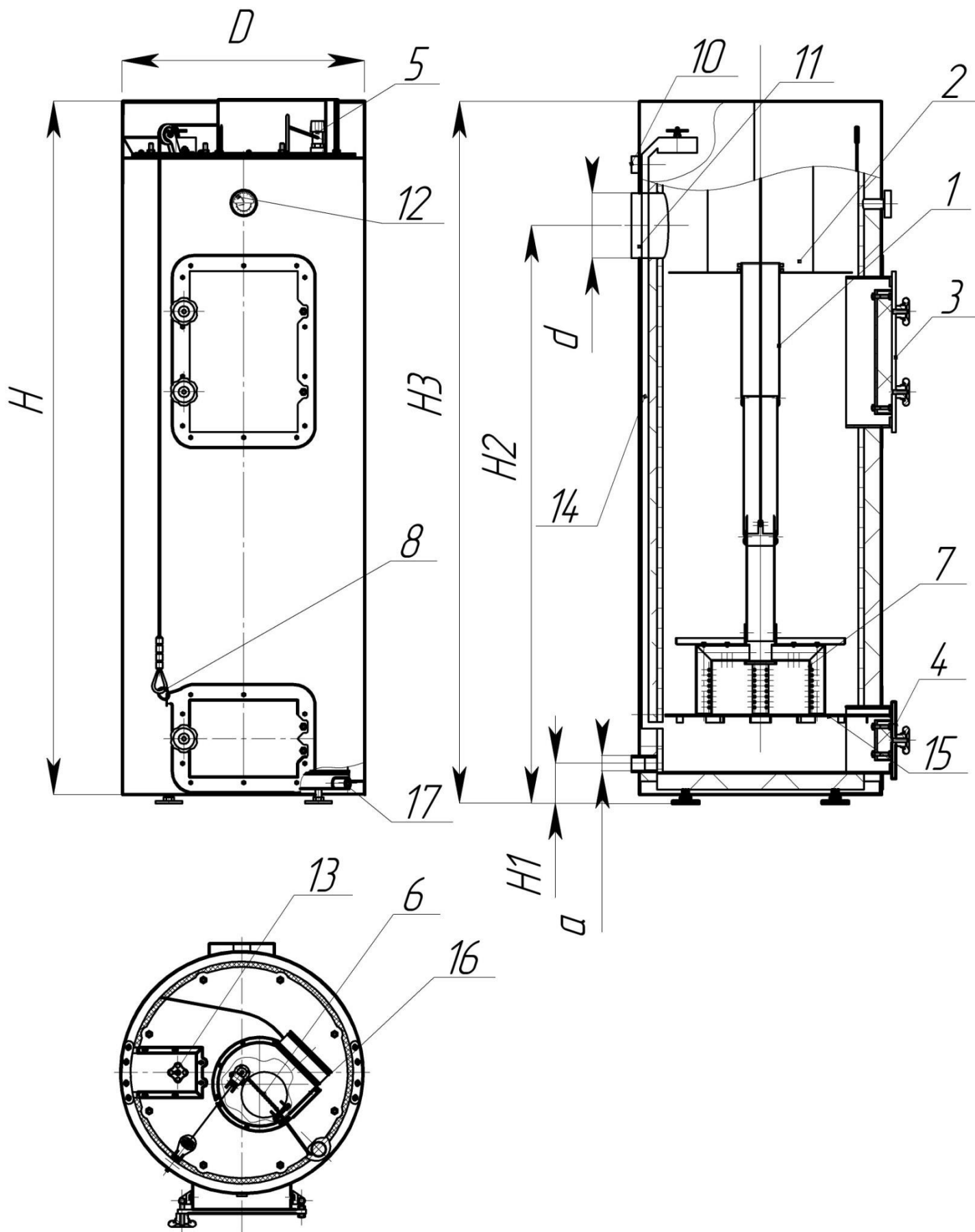
Рис. 2. Габаритные и присоединительные размеры универсальной версии Comfort-XXG. 1.7. УСТРОЙСТВО И ПРИНЦИП РАБОТЫ
